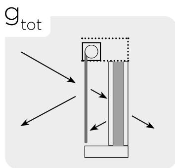
TRANSMITANCIA ENERGÍA SOLAR TOTAL g_{tot} | Transmitância energia solar g_{tot}
