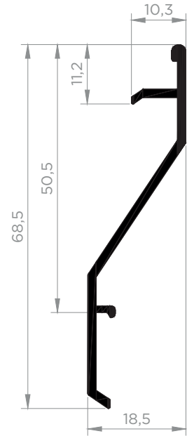
Lama Lâmina | Lamelle | Slat
