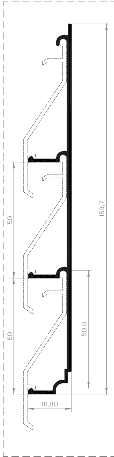
Detalle Pormenor | Détail | Detail
